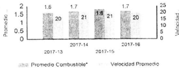
(Km/Litro) vs Velocidad promedio (Km/h)
